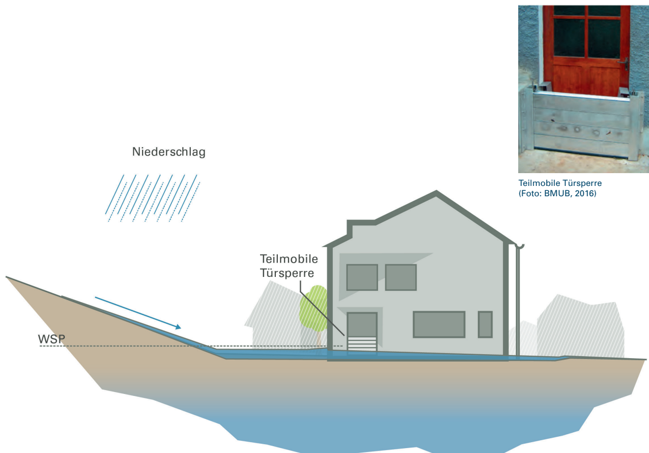
Abbildung 23 Skizze zu möglichen mobilen Türsperrungen (Ingenieurbüro Reinhard Beck)
